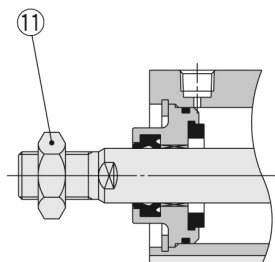
Tige filetée
