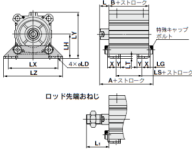
フート形／CQ2L-CDQ2L
