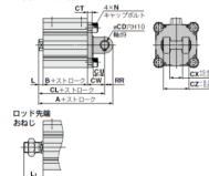
二山クレビス形/CQ2D・CDQ2D
