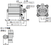
二山クレス形/CQ2D・CDQ2D
