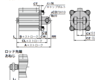
二山クレビス形/CQ2D・CDQ2D
