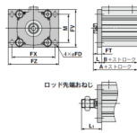
ロッド側フランジ形 / CQ2F-CDQ2F
