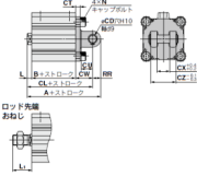
ロッド先端 おねじ
