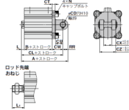
二山クレビス形/CG2D-CDQ2D
