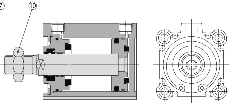
Kolbenstangen-Außengewinde
