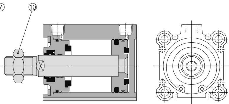
Kolbenstangen-Außengewinde
