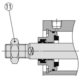
Kolbenstangen-Außengewinde
