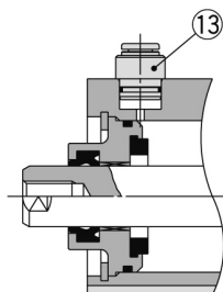
mit Steckverbindung
