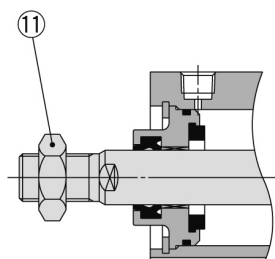
Kolbenstangen-Außengewinde
