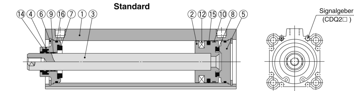
Kolbenstangen-Außengewinde
