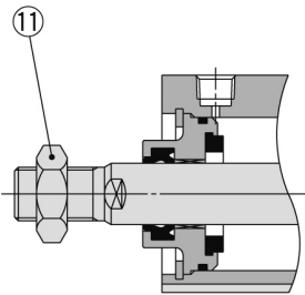
Kolbenstangen-Außengewinde
