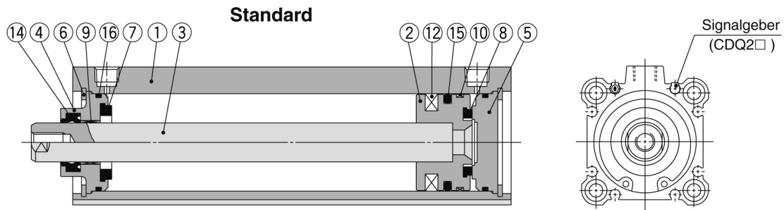
Kolbenstangen-Außengewinde
