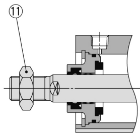
Kolbenstangen-Außengewinde
