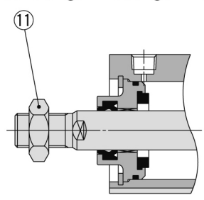
Kolbenstangen-Außengewinde
