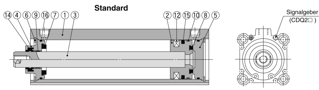
Kolbenstangen-Außengewinde
