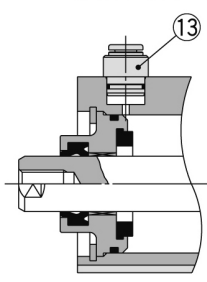
mit Steckverbindung
