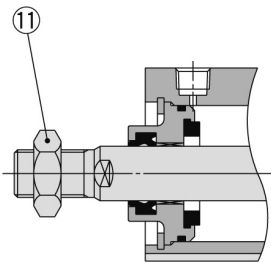
Kolbenstangen-Außengewinde
