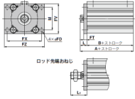
ロッド端フランジ形/CDQ2F
