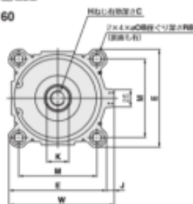
通し穴／C型Q2B ø125～ø160
