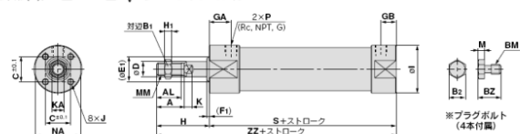
基本形(B)/C□G5B A A □S R V : エアクション付
