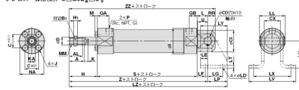
クレビスー体形(E)/C□G5E N A □S R V
