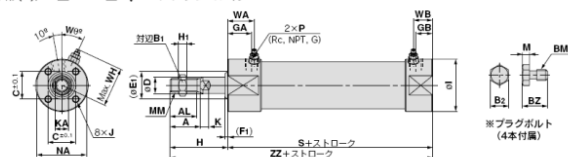
基本形(B)/C□G5B A A □S R V : エアクション付
