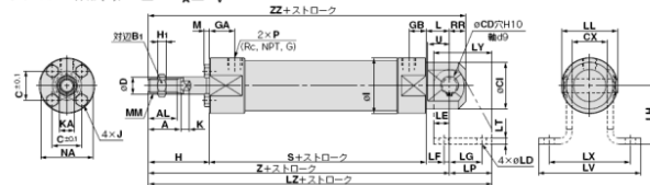
クレビスー体系(E)/C□G5E N A □S R V
