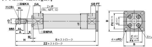
ヘッド側フランジ形(G)/C□G5G A N □S V R
