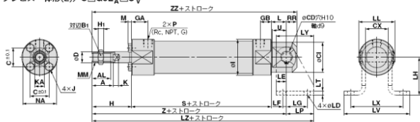
クレビス一体形(E)/C□G5E N A □S R V
