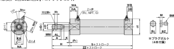
基本形(B)/C□G5BA□S V R :エアクッション付
