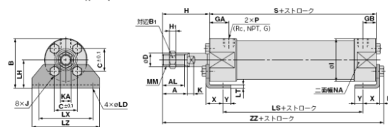
軸方向フート形(L)/C□G5L N A □S R V
