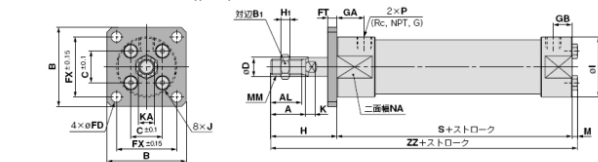
ロッド側フランジ形(F)/C□G5F N A □S R V
