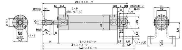
クレビスー体形(E)/C□G5E A N □S V R
