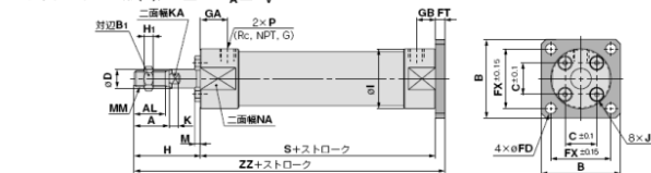
ヘッド側フランジ形(G)/C□G5G A N □S V R
