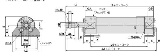
軸方向フート形(L)/C□G5L A N □S V R
