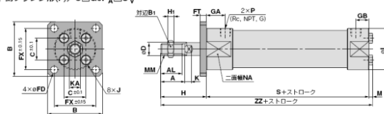
ロッド側フランジ形(F)/C□G5F A N □S V R
