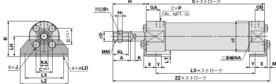
軸方向フート形(L) / C□G5L N □S R V
