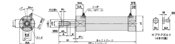
基本形(B) / C□G5BA□S R V : エアアクション付
