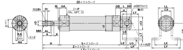
クレビスー体形(E) / C□G5E N □S R V
