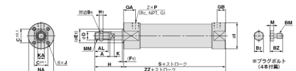
基本形(B) / C□G5BA□S R V : エアアクション付
