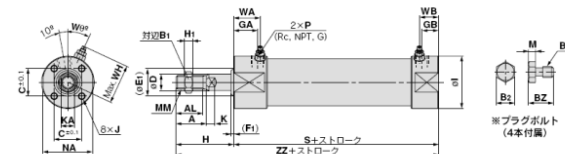
基本形(B)/C□G5B A A □S R V : エアクッション付
