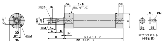
基本形(B)/C□G5B A A □S R V : エアクッション付
