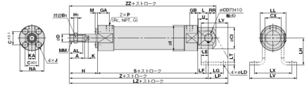
クレビスー体形(E)/C□G5E N A □S R V
