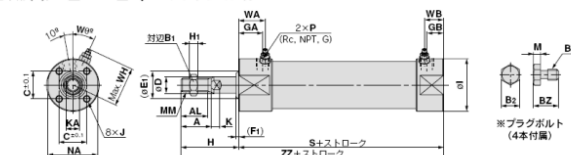
基本形(B)/C□G5BA□S V R : エアアクション付
