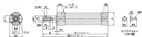
基本形(B)/C□G5BA□S V R : エアアクション付
