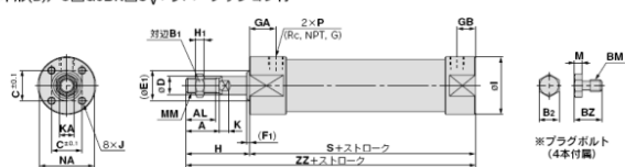
基本形(B)/C□G5BA N A □S R V : エアクッション付
