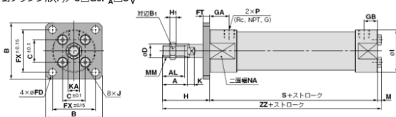
ロッド側フランジ形(F)/C□G5F N □S R V
