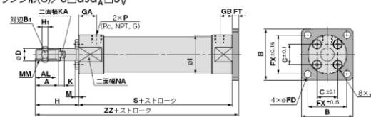
ヘッド側フランジ形(G)/C□G5G N □S R V
