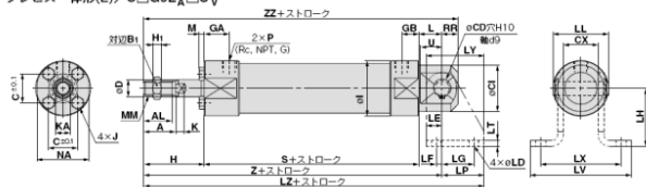
クレビスー体形(E)/C□G5E N □S R V
