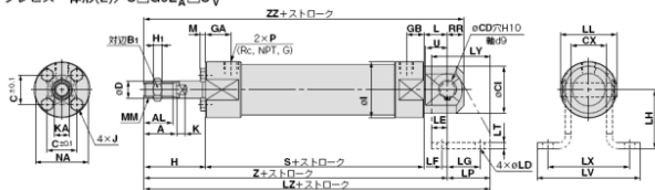
クレビス型形(E)/C□G5E N A □S R V
