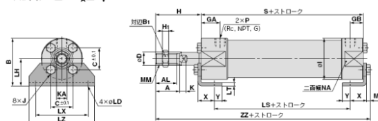
軸方向フート形(L)/C□G5L A N □S V R
