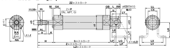
クレープシーテ形(E)/C□G5E N A □S R V
