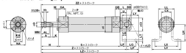
クレープシー一体形(E)/C□G5E□S R V
