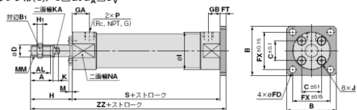
ヘッド側フランジ形(G)/C□G5G N □S V R
