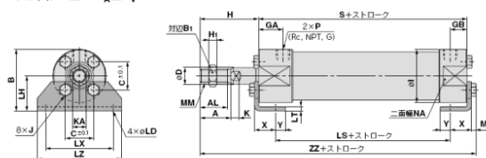
軸方向フート形(L)/C□G5L N □S V R
