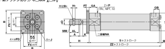
ロッド側フランジ形(F)/C□G5F N □S R A V
