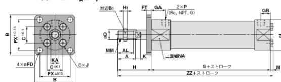
ロッド側フランジ形(F) / C□G5F N □S R V
