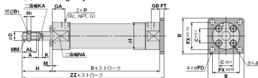
ヘッド側フランジ形(G) / C□G5G N □S R V
