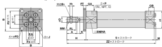
ロッド側フランジ形(F)/C□G5FA N □S R V
