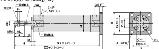
ヘッド側フランジ形(G)/C□G5GA N □S R V
