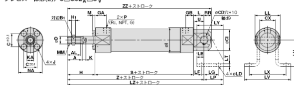
クレブスー体形(E)/C□G5E N □S R V
