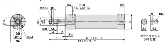
基本形(B)/C□G5BA□S R V : エアクション付
