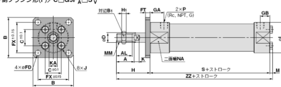
ロッド側フランジ形(F)/C□G5F N A □S R V
