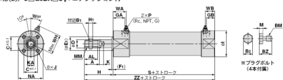
基本形(B)/C□G5BA□S R V : エアクッション付
