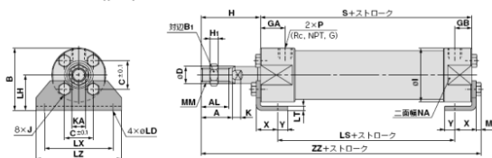
軸方向フート形(L)/C□G5L N □S V R
