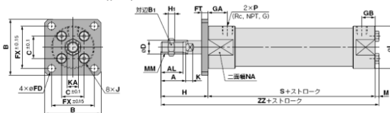
ロッド側フランジ形(F)/C□G5F N □S V R
