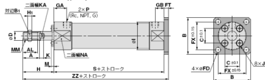
ヘッド側フランジ形(G)/C□G5G N □S V R
