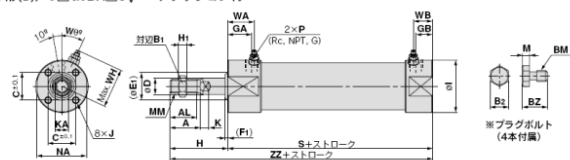
基本形(B)/C□G5BA□S R V : エアクション付
