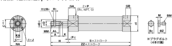
基本形(B)/C□G5BA□S R V : エアクション付
