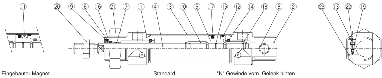
Eingebauter Magnet
