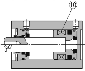
mit Signalgeber (eingebauter Magnetring)
