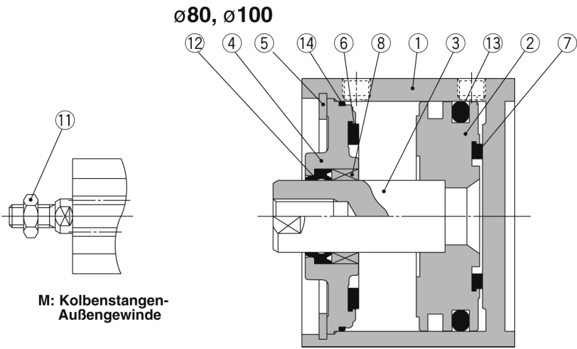
mit Signalgeber (eingebauter Magnetring)
