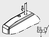
MONOSTABILE BETÄTIGUNG ANSCHLUSS 2 druckluftunterstützt
