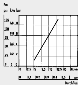
Minimaldurchfluss-Diagramm SY1
