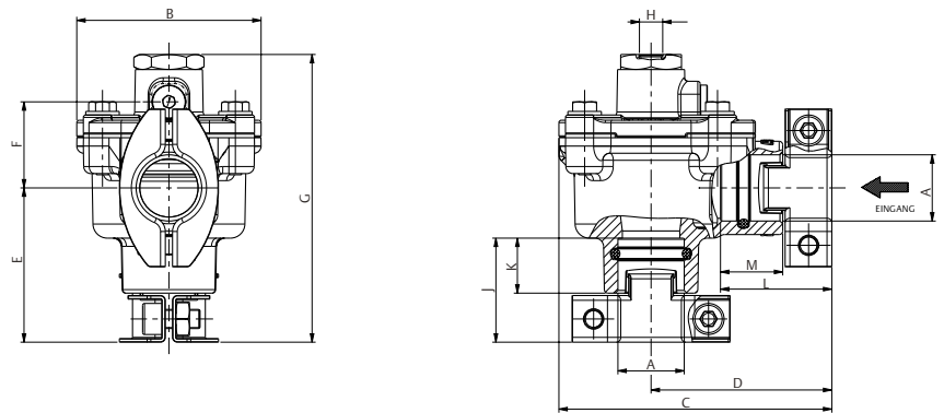
Abb. 2: Mit externer Vorsteuerung
