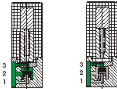
Stellung 1 (Ruhestellung)
